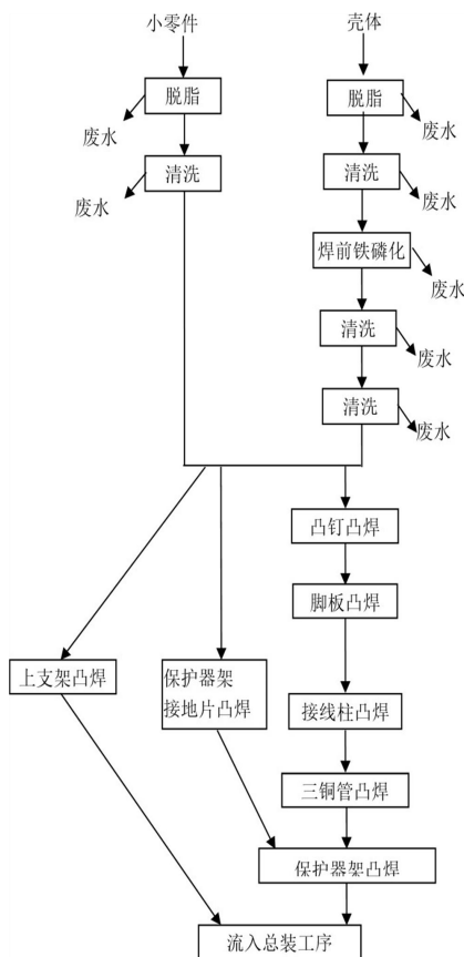
图 2.5-2 企业下壳体组件工艺流程及污染物产生示意图
