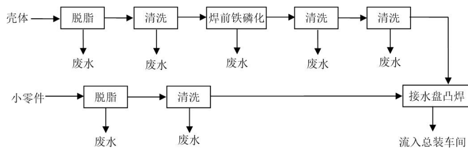
图 2.5-1 企业上壳体组件生产工艺流程及污染物产生示意图
