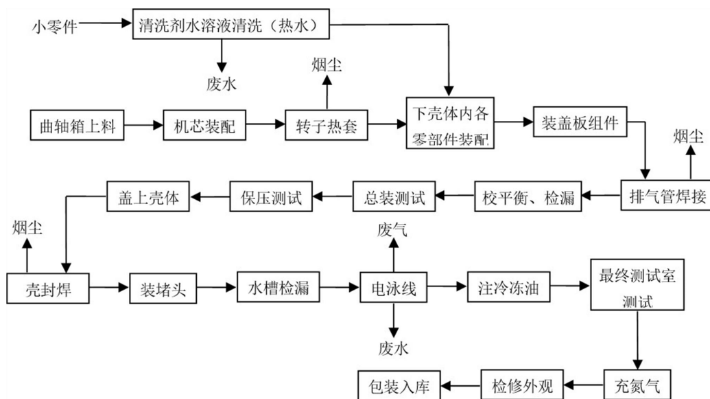
图 2.5-9 企业压缩机总装实际生产工艺及污染物产生示意图
