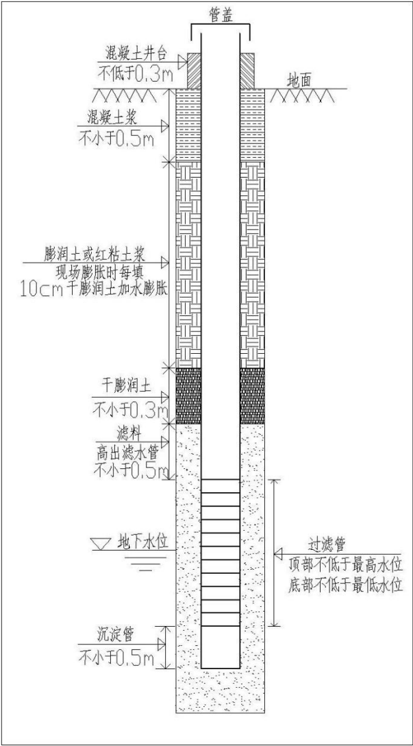
图 7-1 地下水采样井结构示意图
