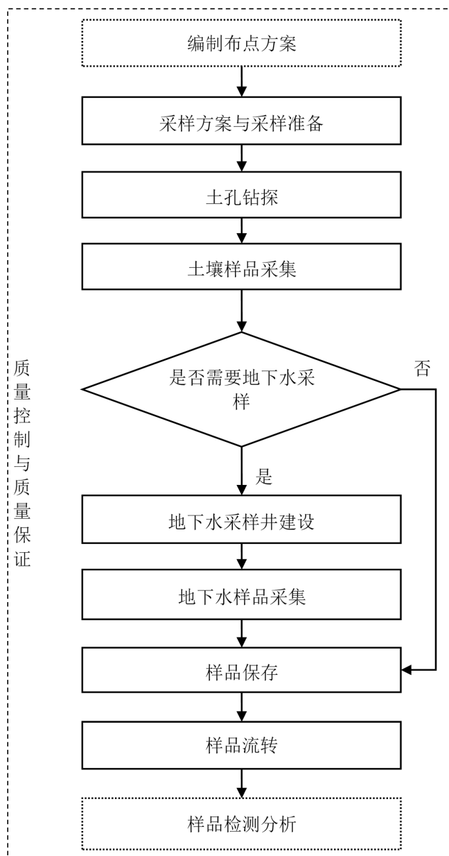
图 1-2 土壤和地下水自行监测现场采样工作程序
