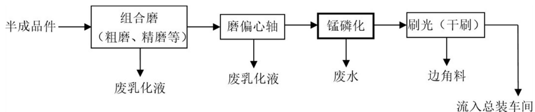
图 2.5-4 曲轴箱生产工艺及污染物产生示意图
