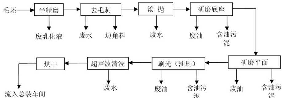
图 2.5-7 阀板实际生产工艺及污染物产生示意图
