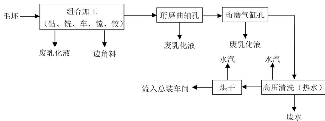
图 2.5-3 曲轴箱生产工艺及污染物产生示意图
