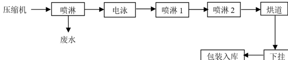
图 2.5-10 电泳线工艺流程及污染物产生示意图
