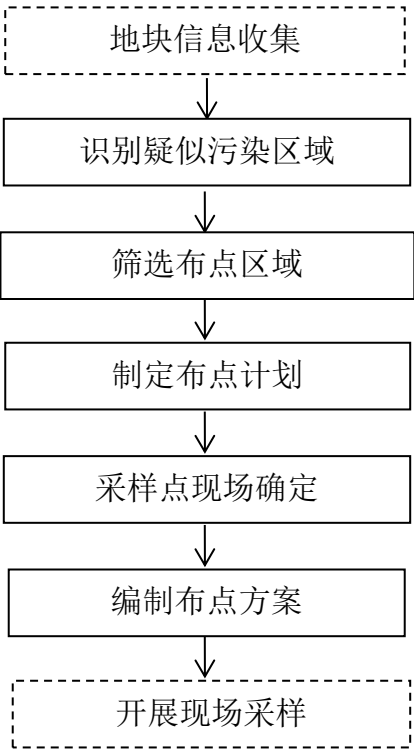
图 1-1 自行监测布点工作程序
