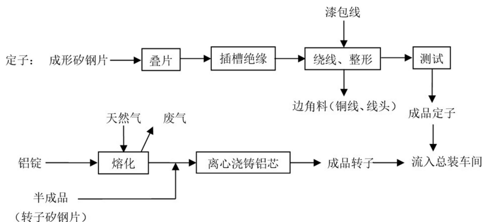
图 2.5-8 转子、定子实际生产工艺及污染物产生示意图
