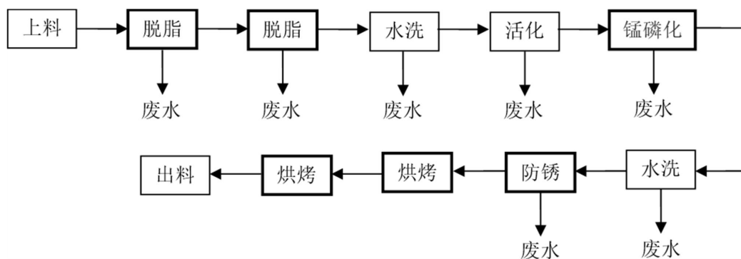
图 2.5-5 锰磷化实际生产工艺及污染物产生示意图
