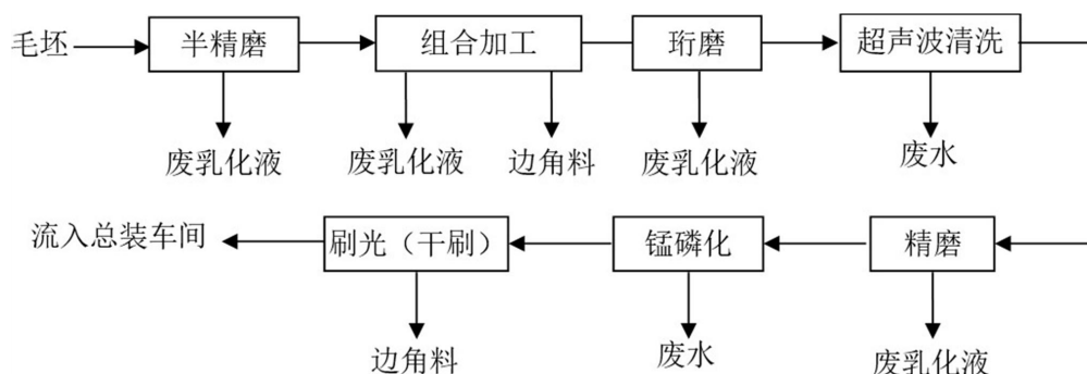
图 2.5-6 活塞实际生产工艺及污染物产生示意图
