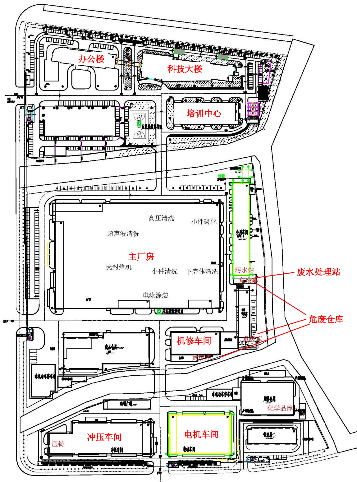
图 2.3-11 企业总平面布置
