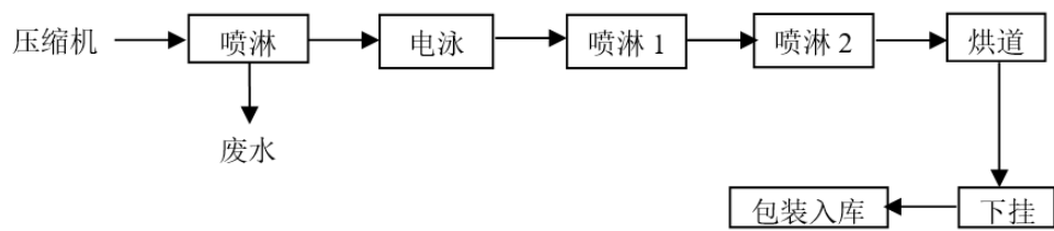
图 2.3-9 企业压缩机总装生产工艺及污染物产生示意图
