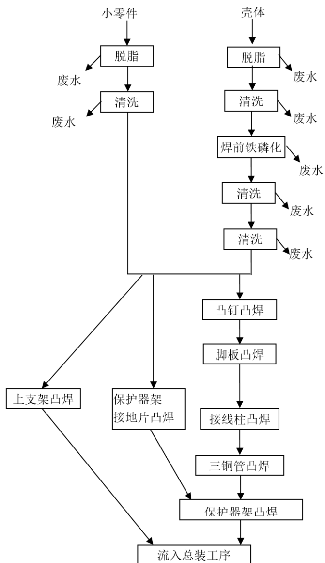
图 2.3-2 企业下壳体组件工艺流程及污染物产生示意图
